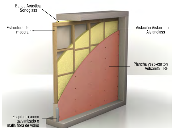
b) Tabique Estructural
